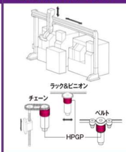
工作機械のガントリーロボット
