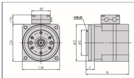
外形寸法
