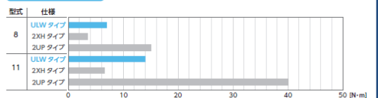
許容モーメント荷重比較
